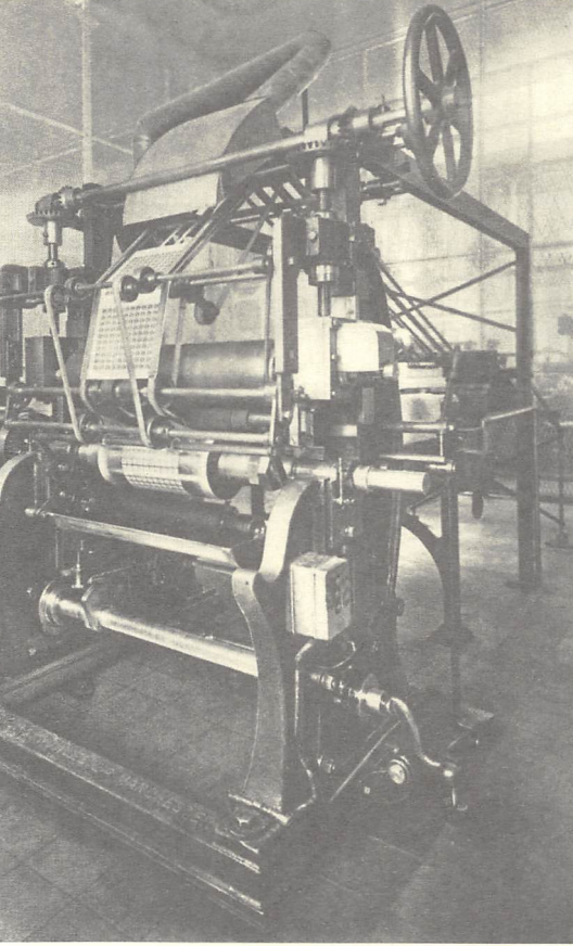
ماكينة للطباعة بطريقة الفوتو جرافير
