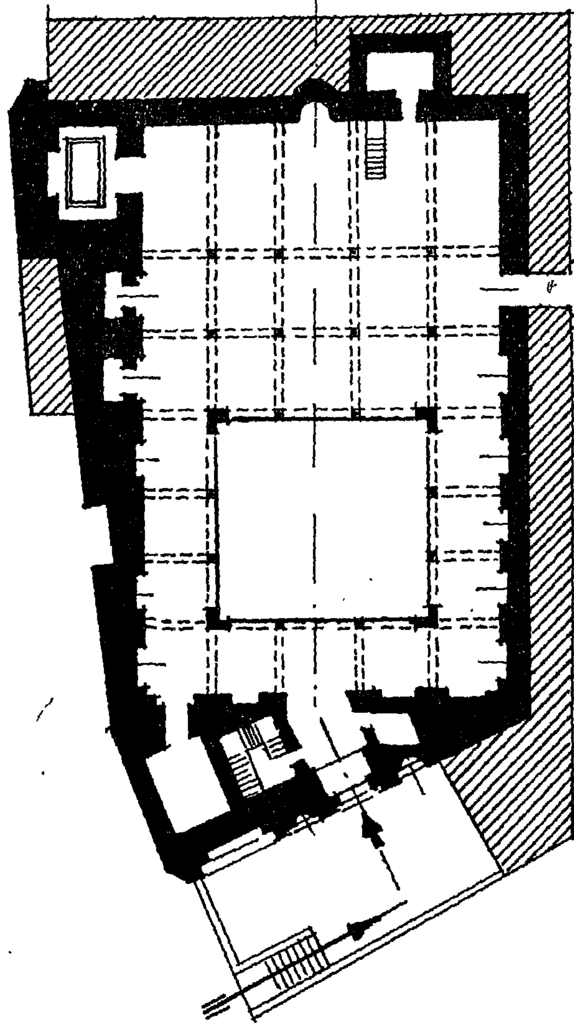
(شكل ٥٢) مسقط أفقى لجامع الأقرم
