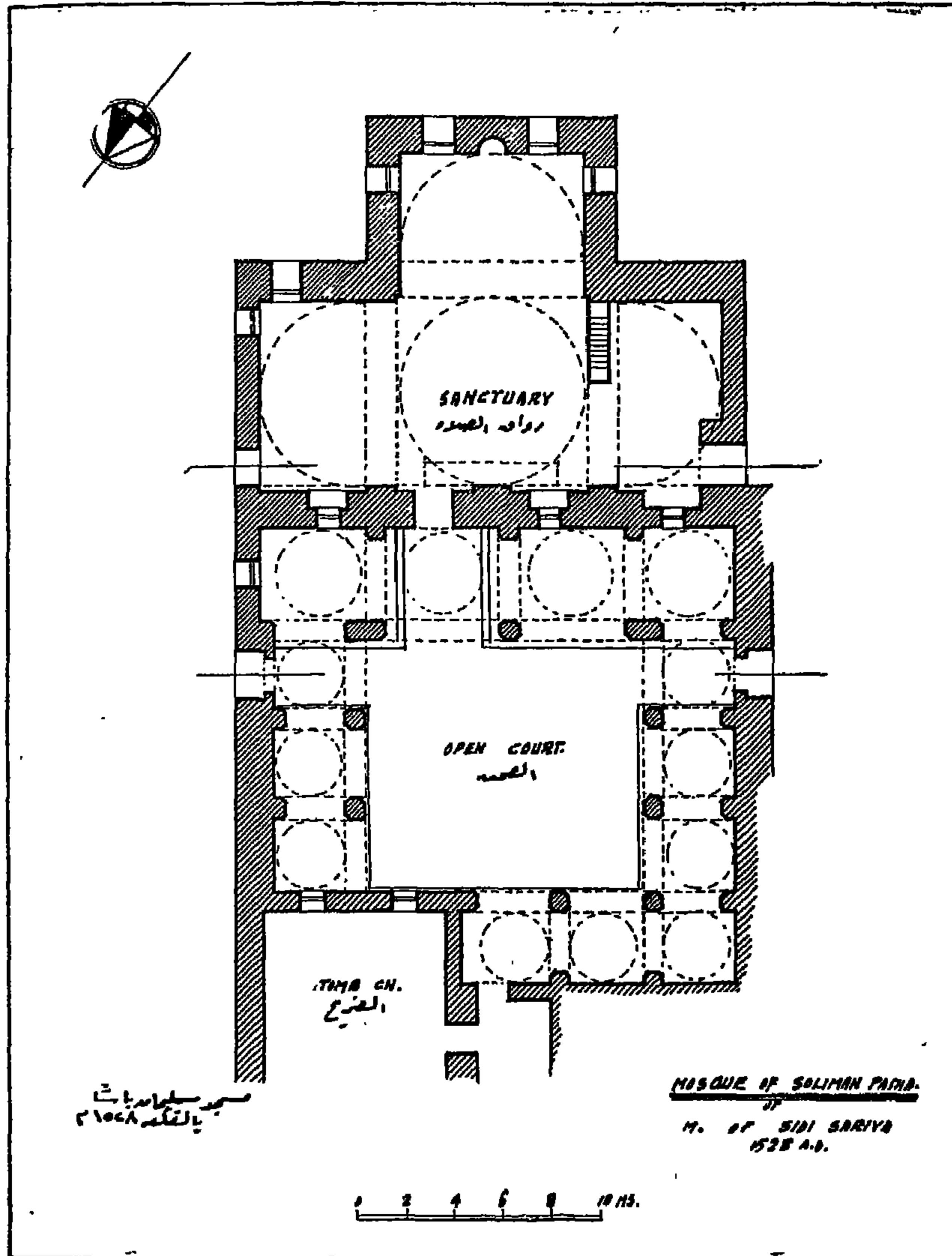
(شكل ٧٧) مسقط أفق لمسجد سليمان باشا بالقاهرة (١٥٢٨ م)
