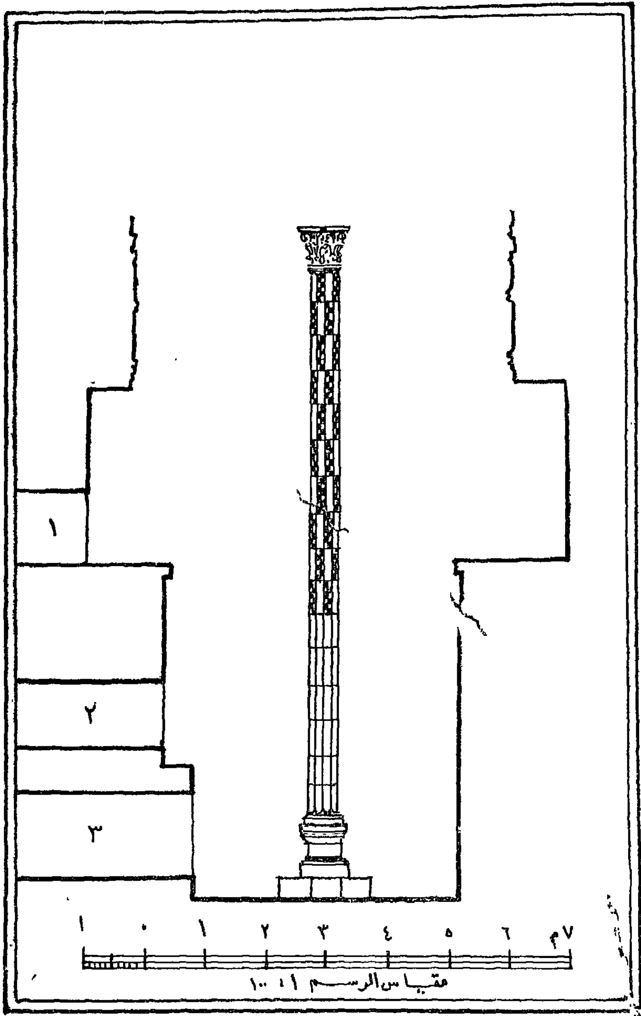
(شكل ٢٢) قطاع في بئر مقياس الروضة
