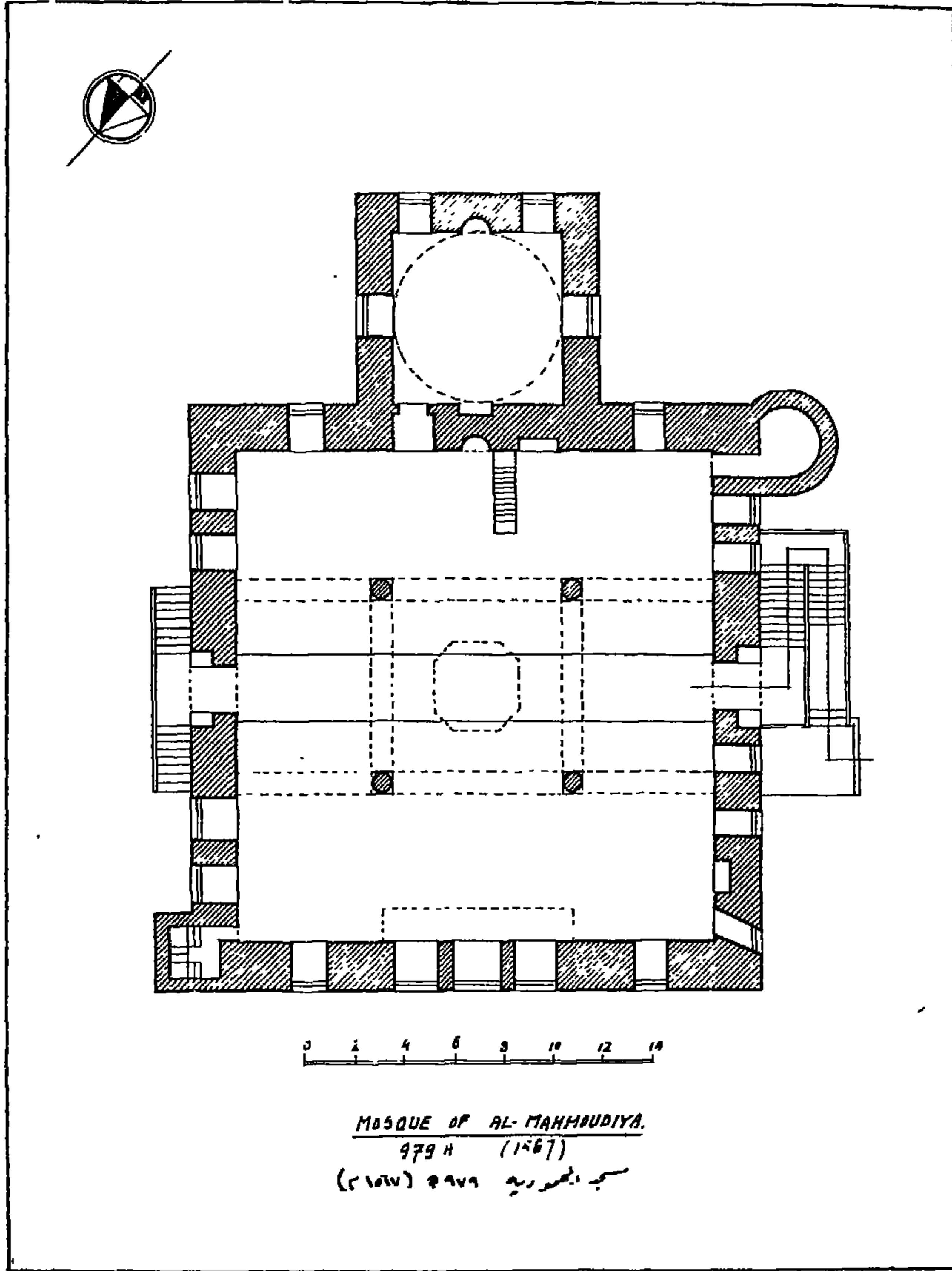
(شكل ٧٨) مسقط أفق لمسجد الحمودية بميدان صلاح الدين بالقلعة (٩٧٩ هـ - ١٥٦٧ م)
