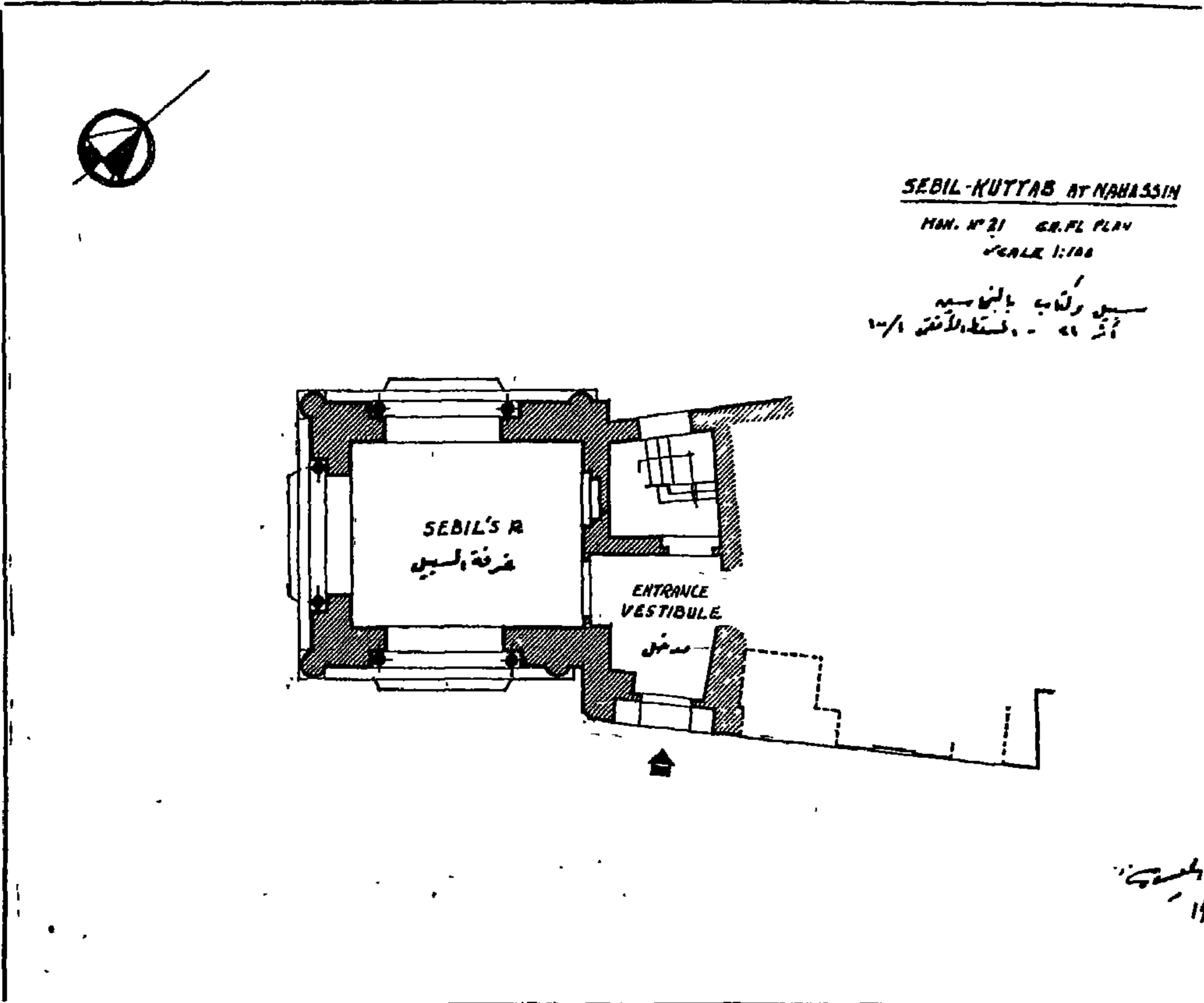
(شكل ٩٠) مسقط الدور الأرضي لسبيل عبد الرحمن كتخدا بالنحاسيين (١٧٤٤ م)
