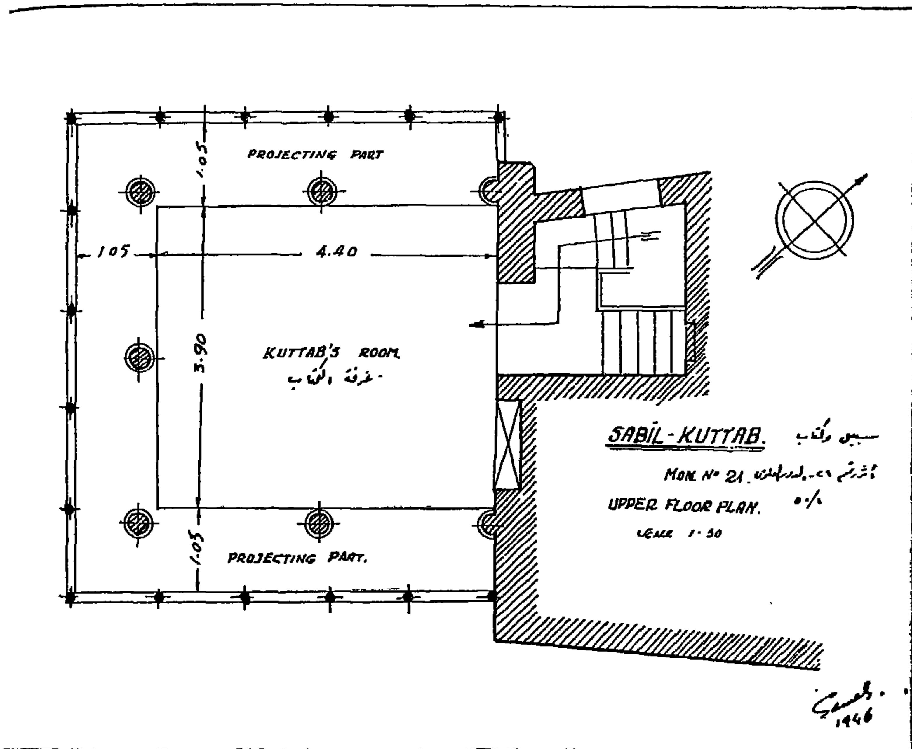
(شكل ٩١) مسقط الدور الأول لسبيل وكتاب عبد الرحمن كتبخدا بالنحاسين (١٧٤٤ م)
