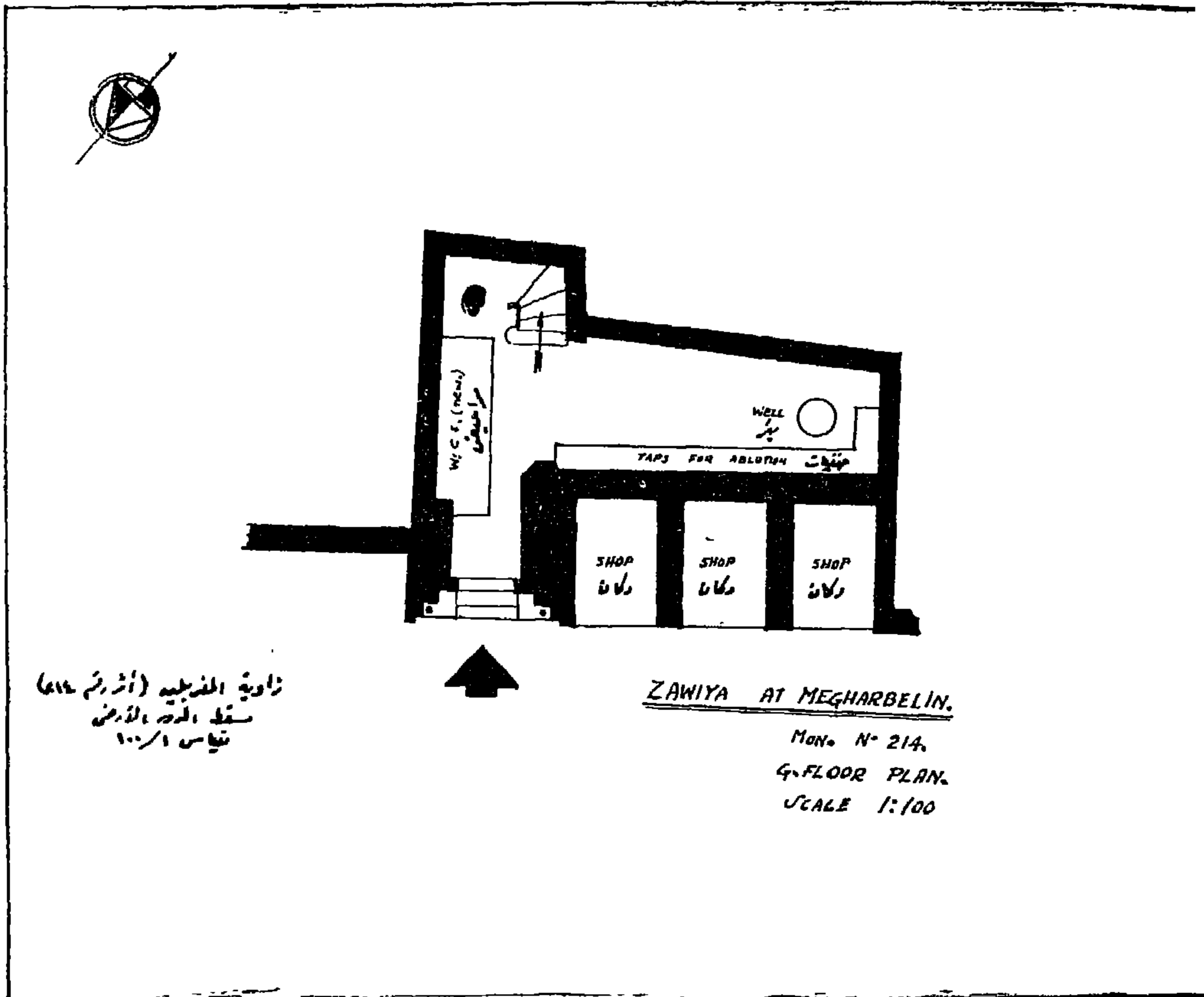
(شكل ٨٧) مسقط الدور الأرضي لزاوية عبد الرحمن كتبخدا بالمغربلين
