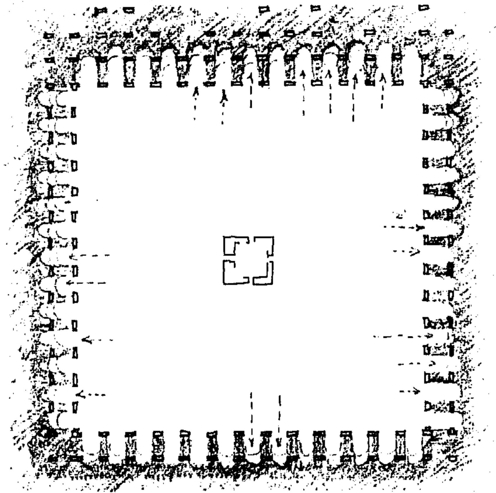
لوحة رقم ١٦٠ رسم يبين تداخل فراغ الصحن في الأقسام المغلفة للمسجد وذلك من خلال الأروقة
