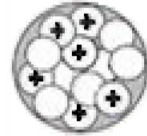
نواه
