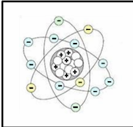
(( مكونات الذرّة ))
