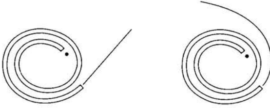
شكل ١: رسم تخطيطي من دراسة مايكل ماكلوسكي (١٩٨٣). ما المسار الذي ستخذه الكرة بعد أن تخرج من المدار الحلزوني؟ (المصدر: ماكلوسكي (١٩٨٣))
