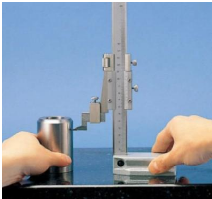
قدمة قياس الارتفاع
