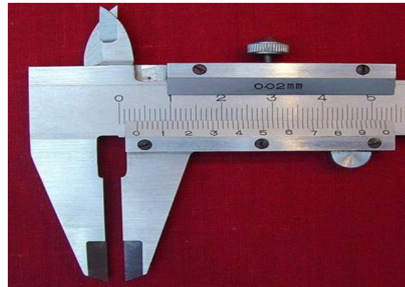
القدمة ذات الورنية العادية
