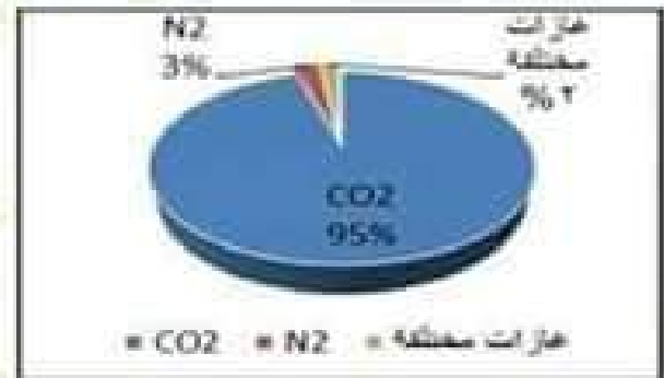
تركيب الغلاف الجوي للمريخ
