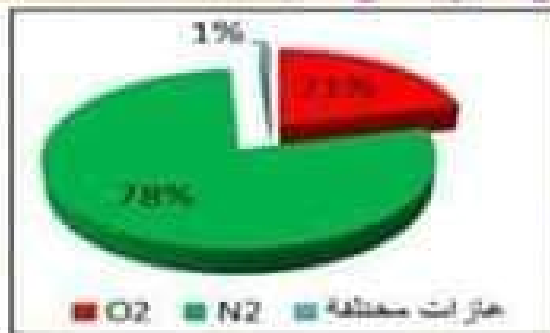
تركيب الغلاف الجوي للأرض
