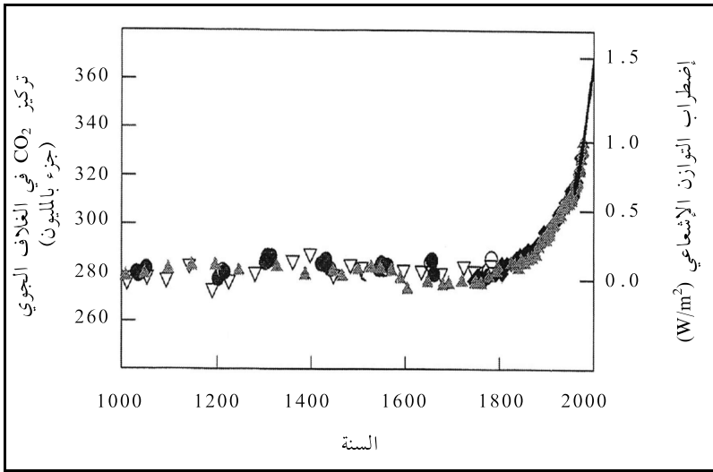
الشكل (3-4): تراكيز غاز CO 2 في الغلاف الجوي
