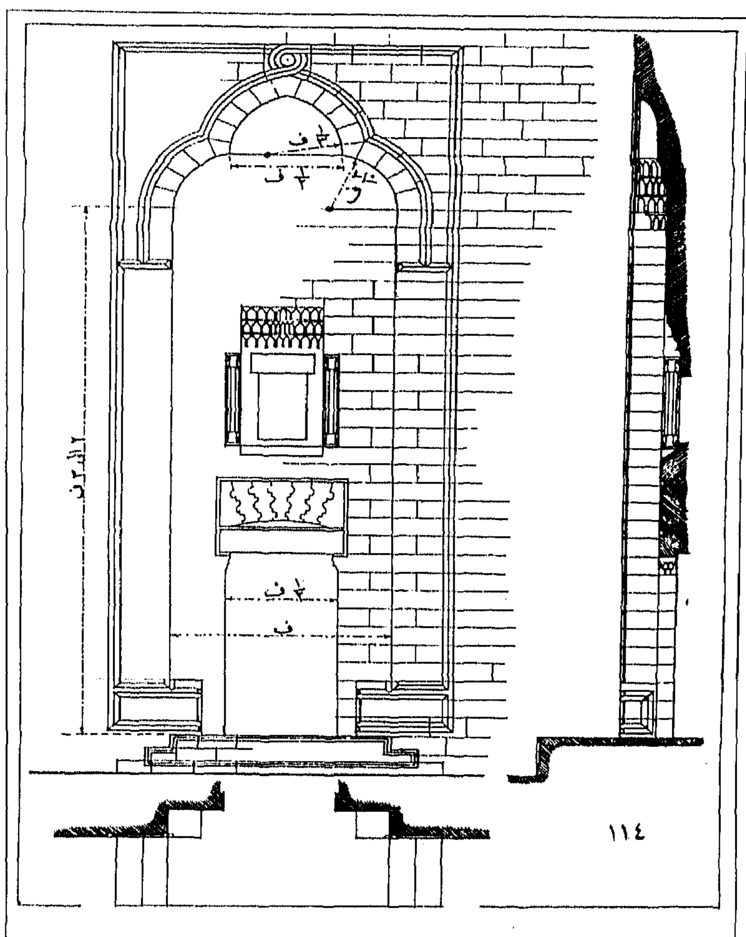
(٧٠) مدخل مملوكي جرکسی (عن ولفرد دल्ली)
