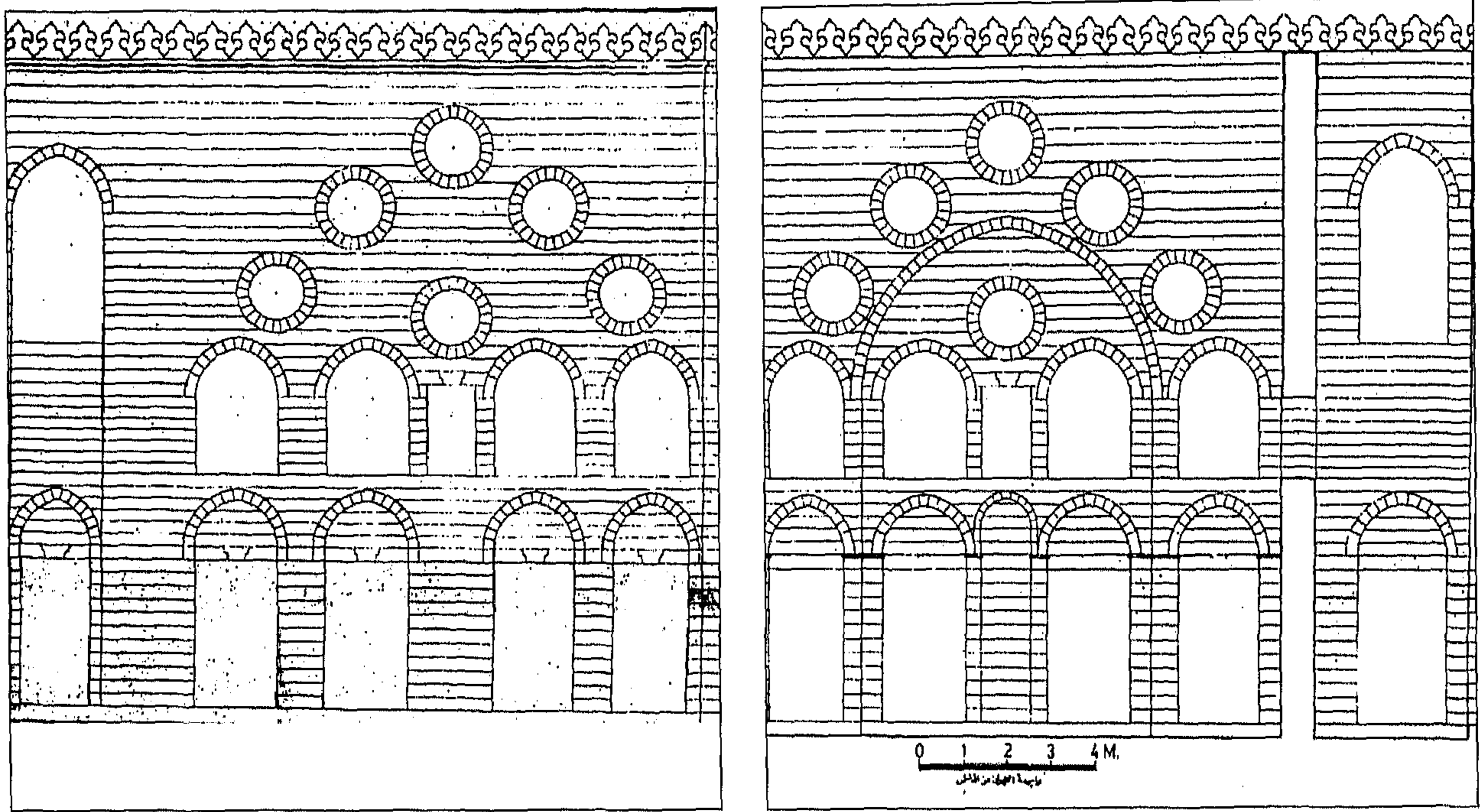
(٢٢) بیمارستان المؤید مشروع إعادة بناء الحائط الغربي
