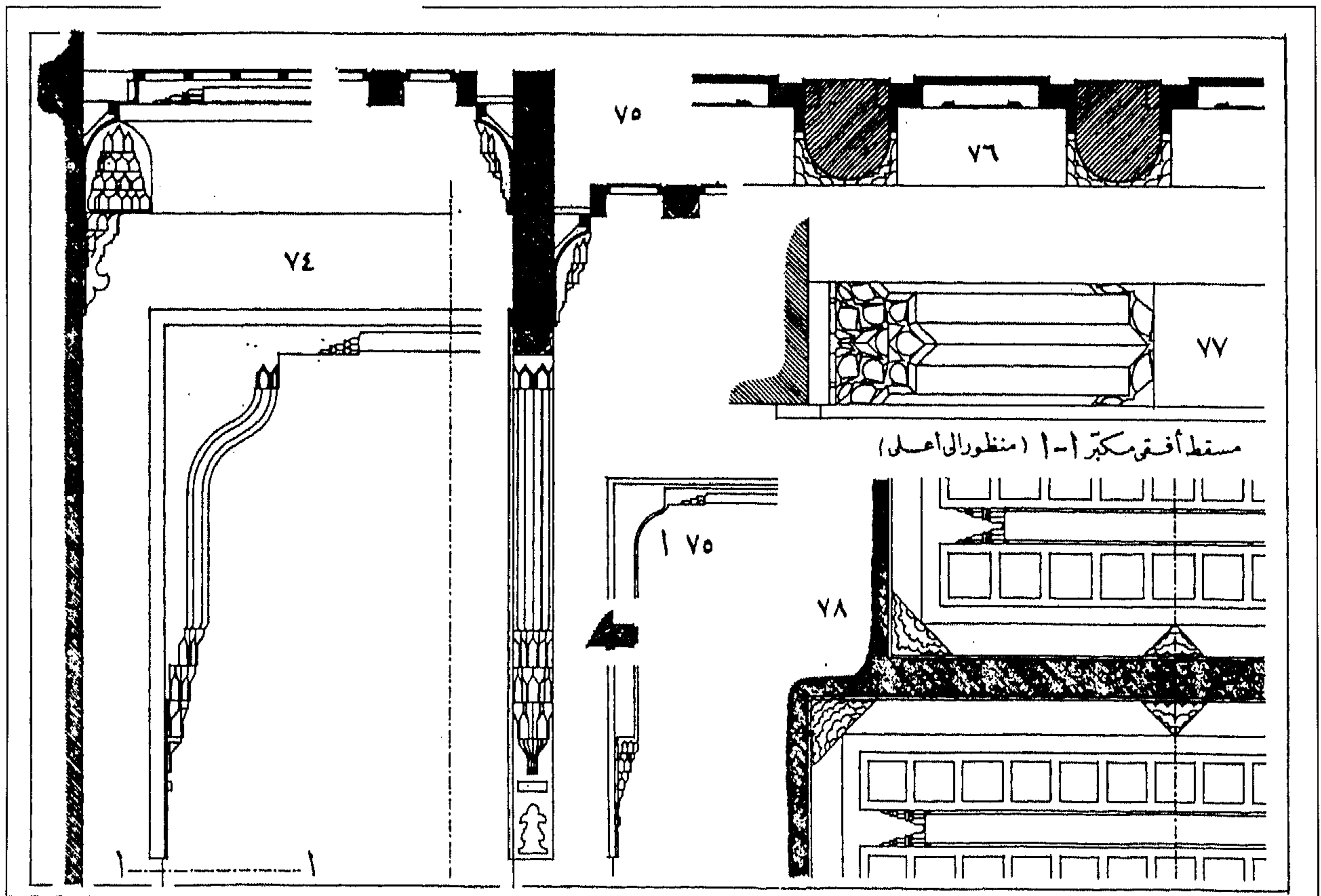
(٧٨) مقرنصات السقوف والبراطيم (عن ولفرد دल्ली)
