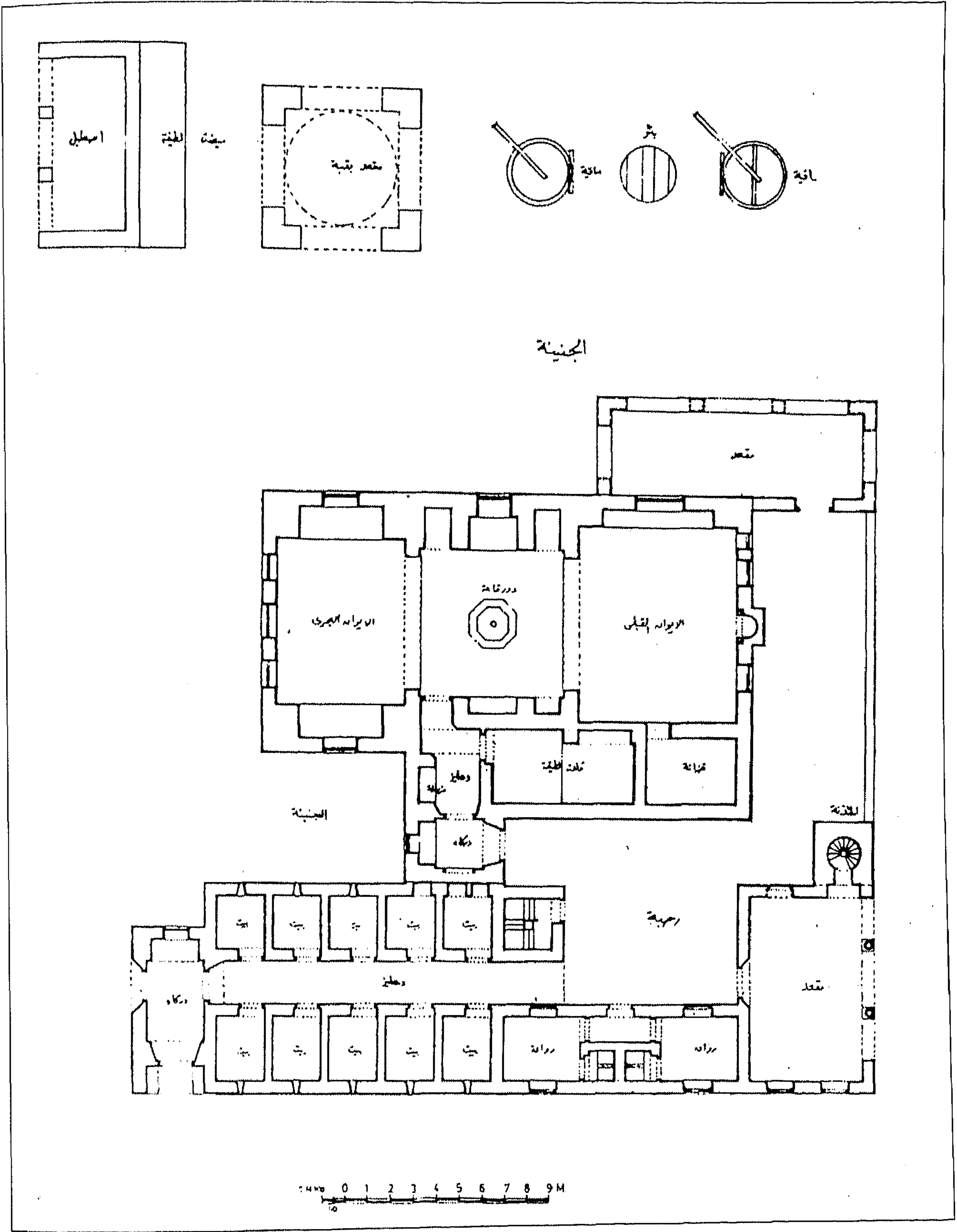
(١٦) خانقاه المؤيد شيخ بالجيزة مسقط أفقى تصويرى لما كانت عليه الخانقاه طبقا لما جاء بوصفها بالوثيقة مقياس الرسم ١ : ١٠٠
