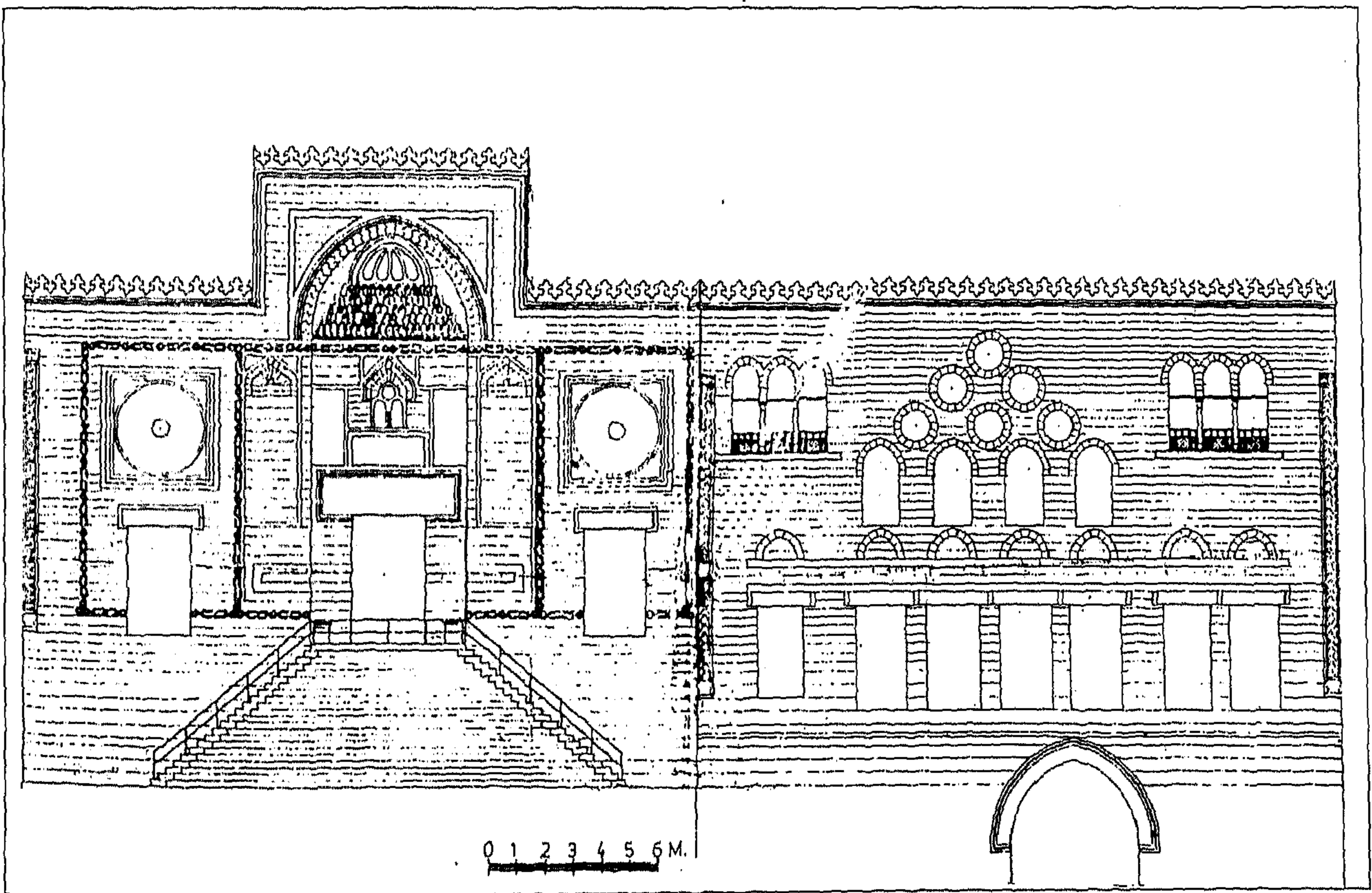
(٢١) بيمارستان المؤيد الواجهة الرئيسية
