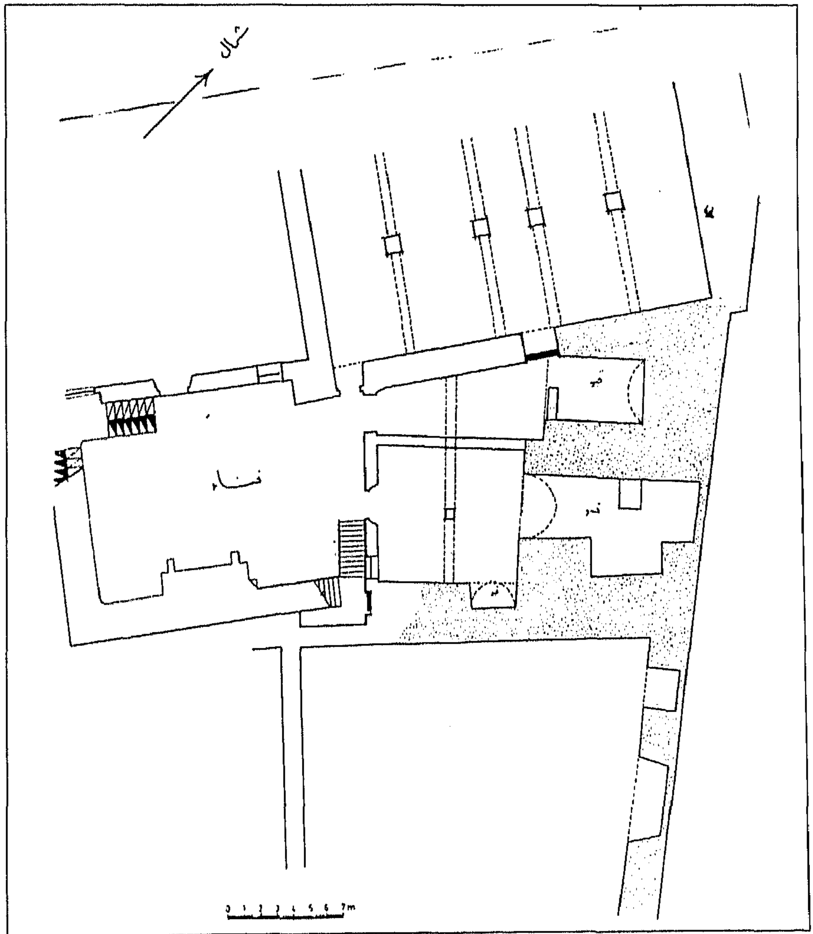
جامع الصوه مسقط أفقى (٧)
