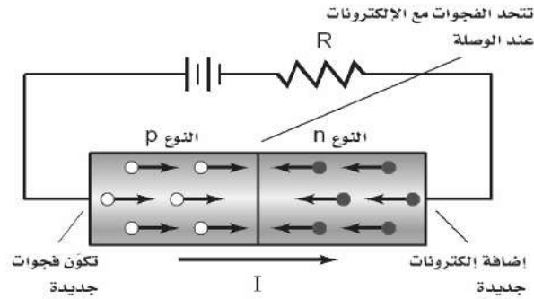
الدايمود المتحيز أمامياً
