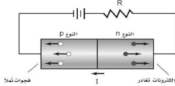
الدايمود المتحيز عكسياً
