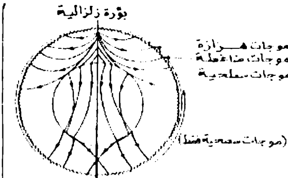
مرور الموجات الزلزالية في طبقات الأرض المختلفة
