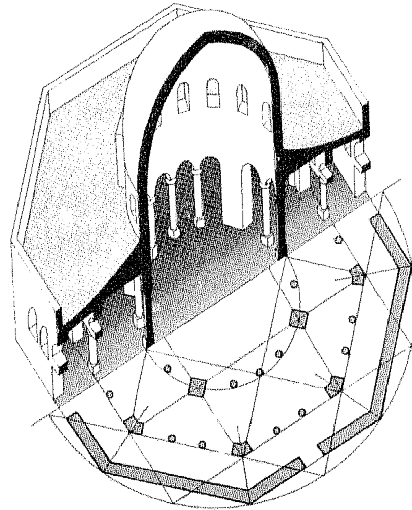
٨ — القدس قبة الصخرة — مقطع منظوري
