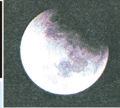
خسوف القمر
