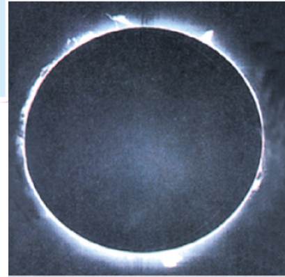
كسوف الشمس
