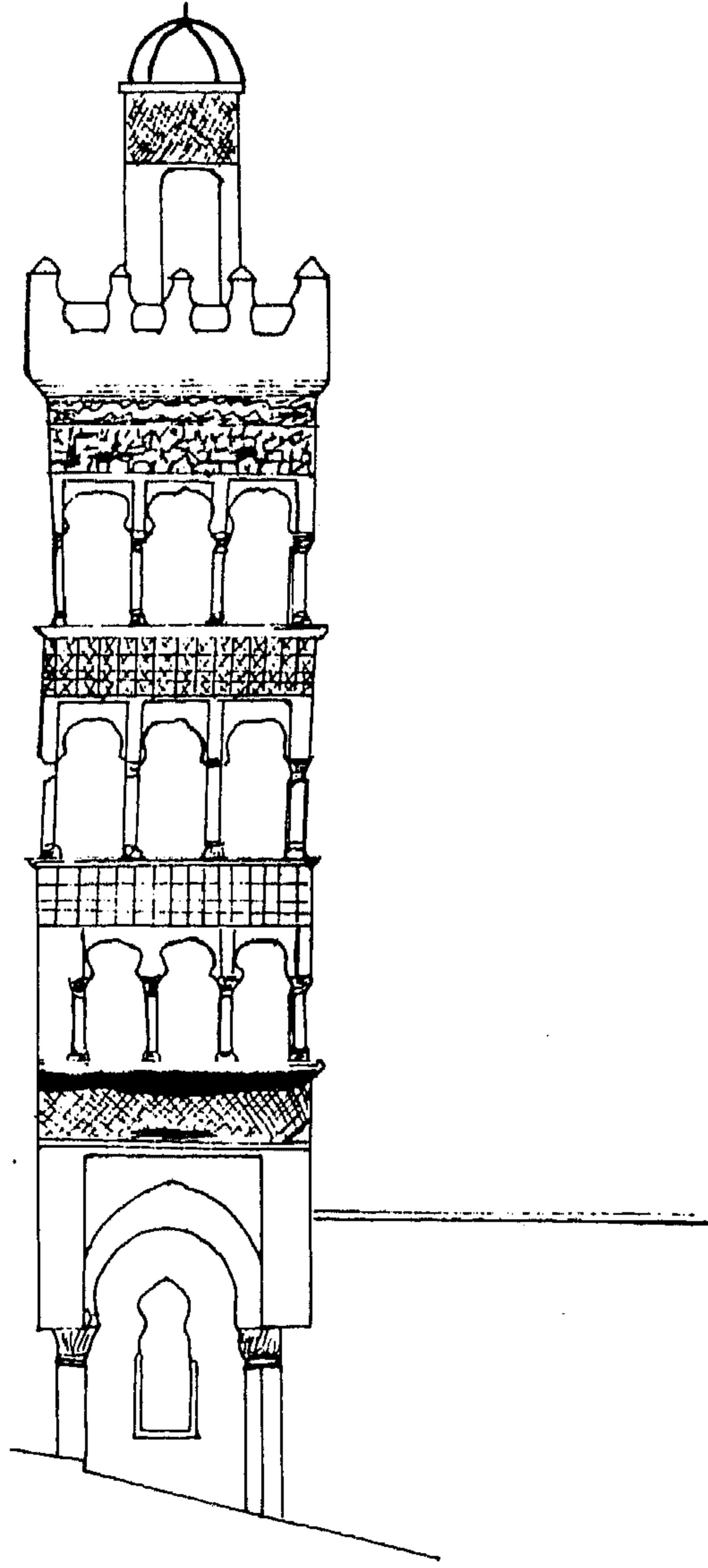
شكل ( ٣٧ ) : واجهة مئذنة مسجد سيدي عبد الرحمن الثعالبي ( الجزائر ) عن ( دوكالسي )
