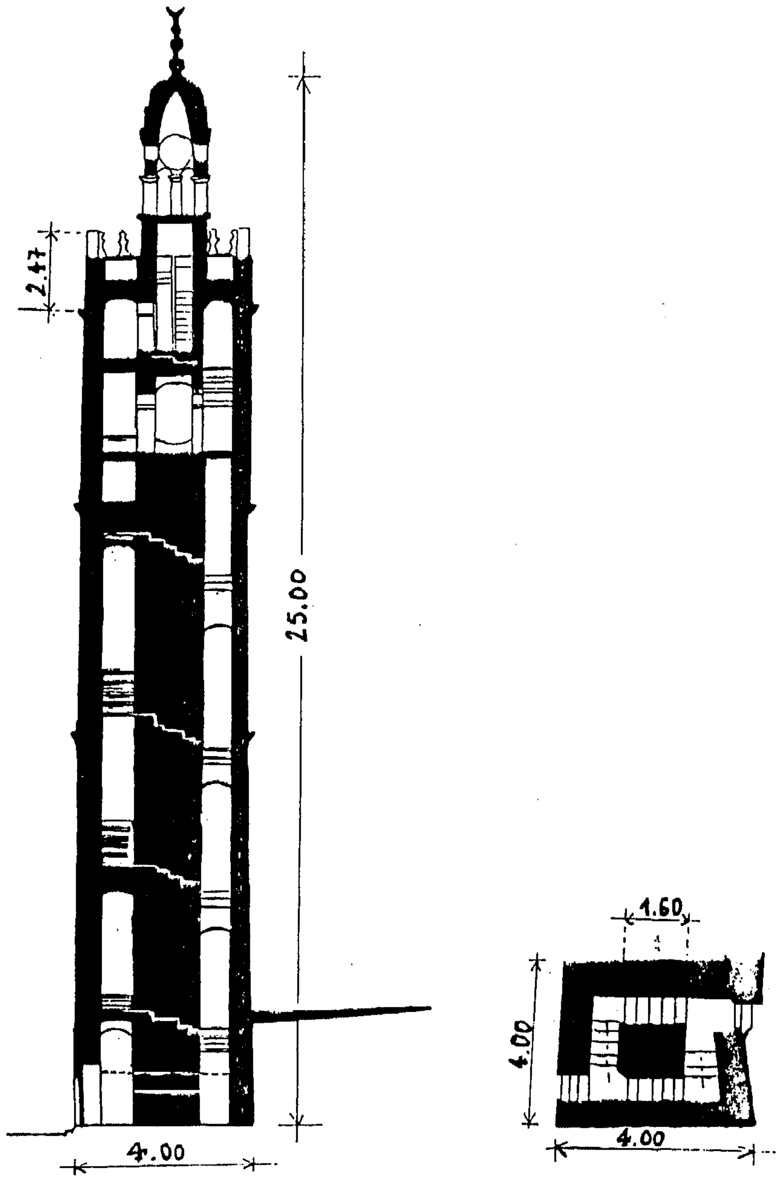
شكل ( ٣٤ ) : مقطع عرضى لمئذنة جامع ( الحواتين ) بالجزائر العاصمة عن ( دوكالى ) بعد التحقيق .
