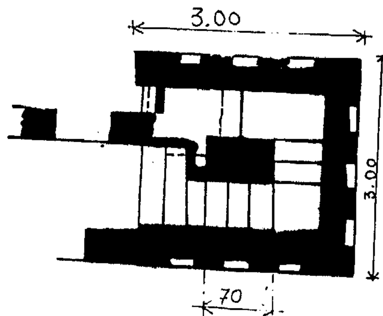
شكل ( ٣٨ ) : مقطع عرضى لمئذنة مسجد سيدي عبدالرحمن الثعالبي - الجزائر عن ( دوکالی ) بعد التحقيق .
