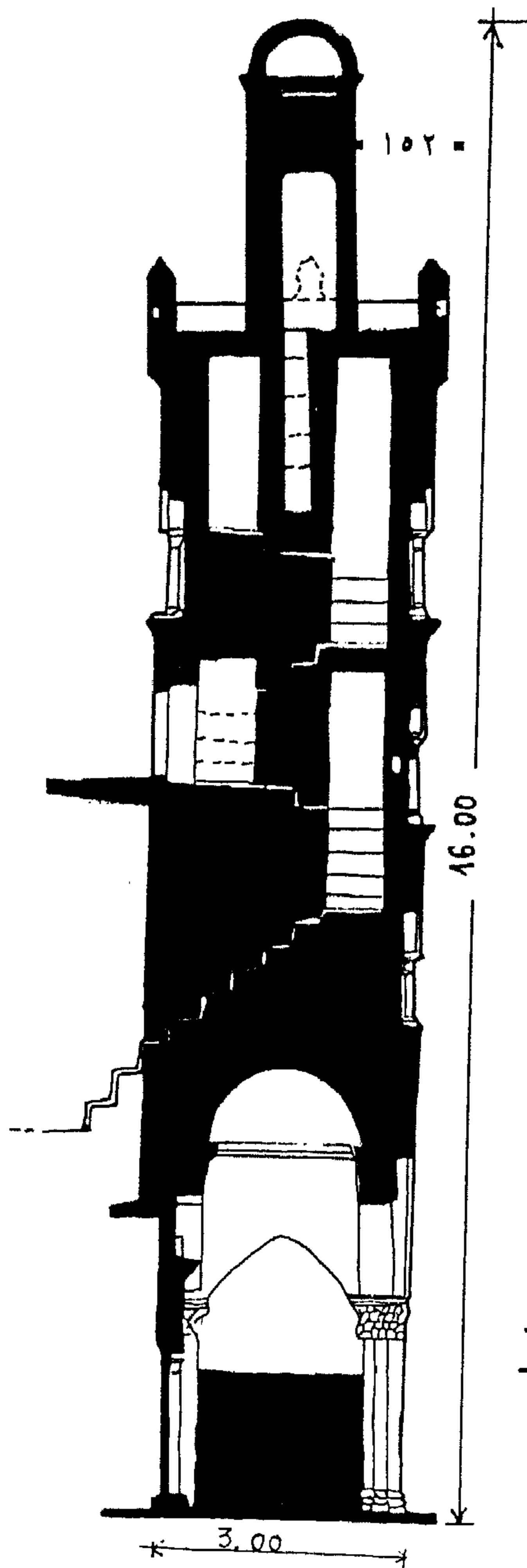
شكل ( ٣٩ ) : مقطع طولى لمئذنة مسجد سيدي عبدالرحمن الثعالبي - الجزائر عن ( دوکالی ) بعد التحقيق .
