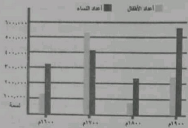
الشكل (٩): شكل لمخطط الأعمدة البياني.
