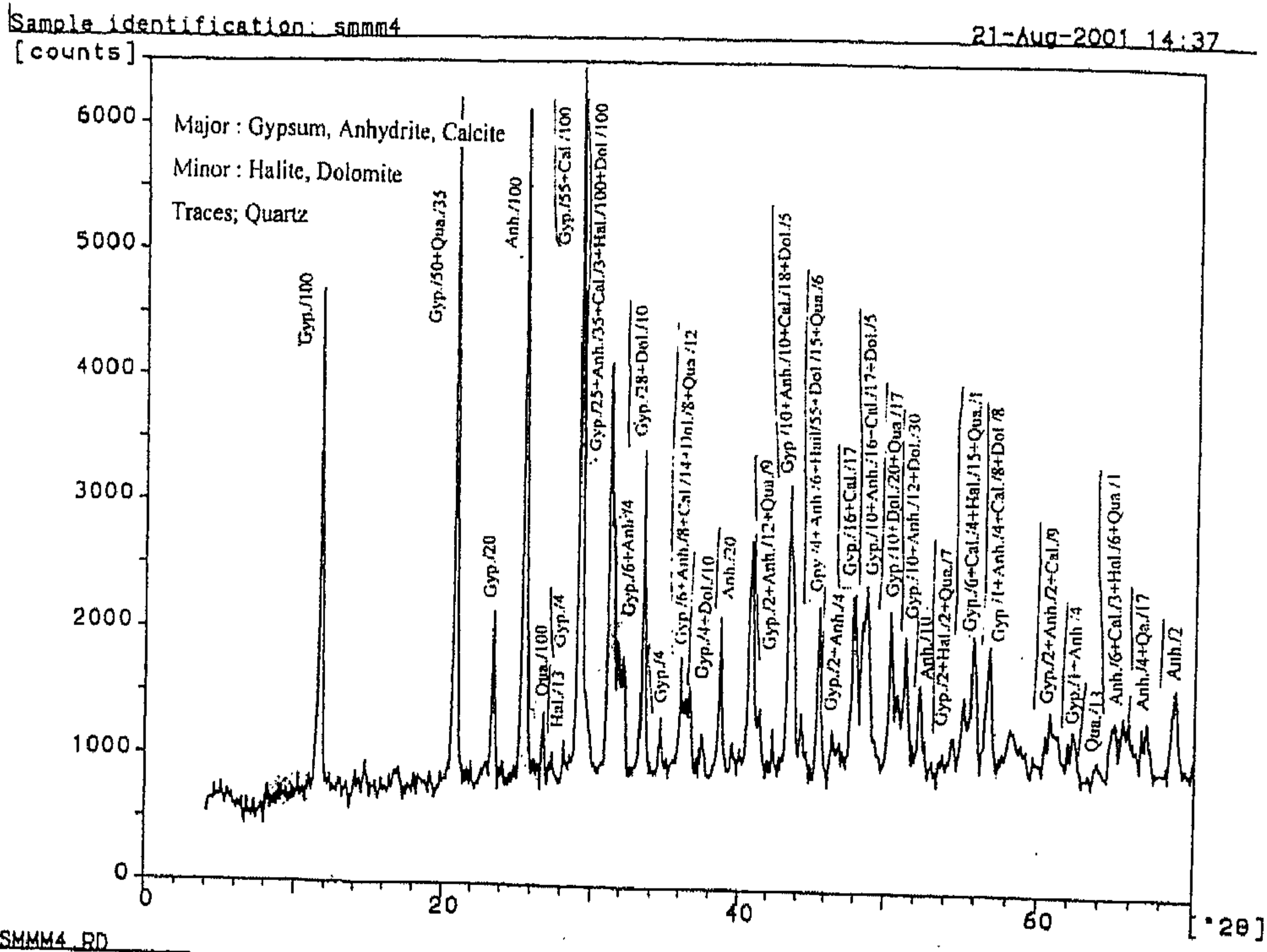
شكل رقم (٣٧) يوضح نمط حيود الأشعة السينية لعينة مونة بناء مثذنة يشبك من مهدى
