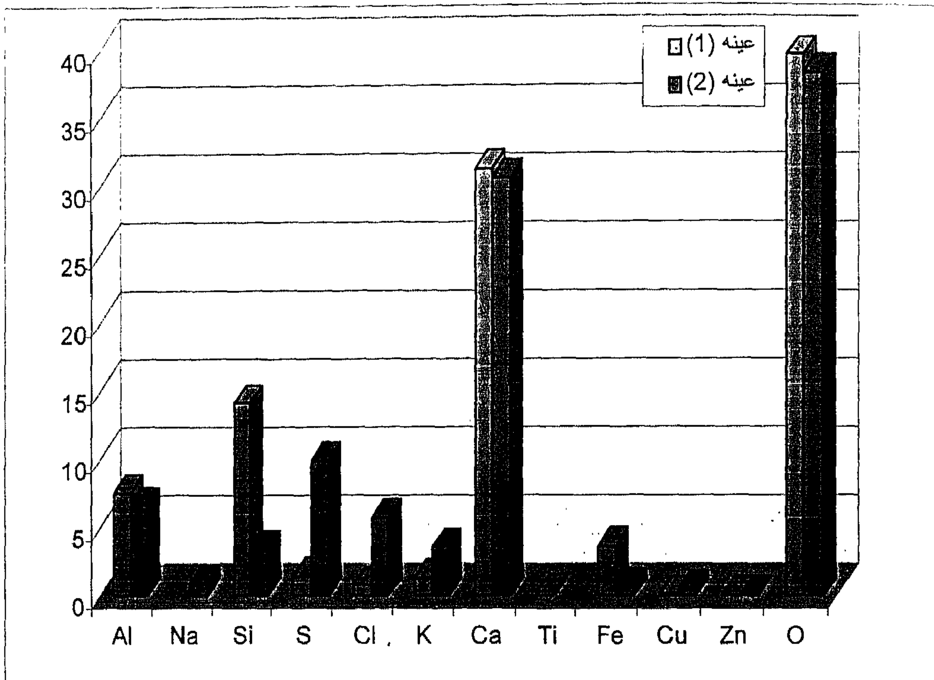
شكل رقم (٣٣) يوضح نسب العناصر بالعينتين رقمي (١)، (٢) من الحجر الجيري بمئذنة يشبك من مهدى واللتين تم تحليلها بواسطة استخدام وحدة [EDX]
