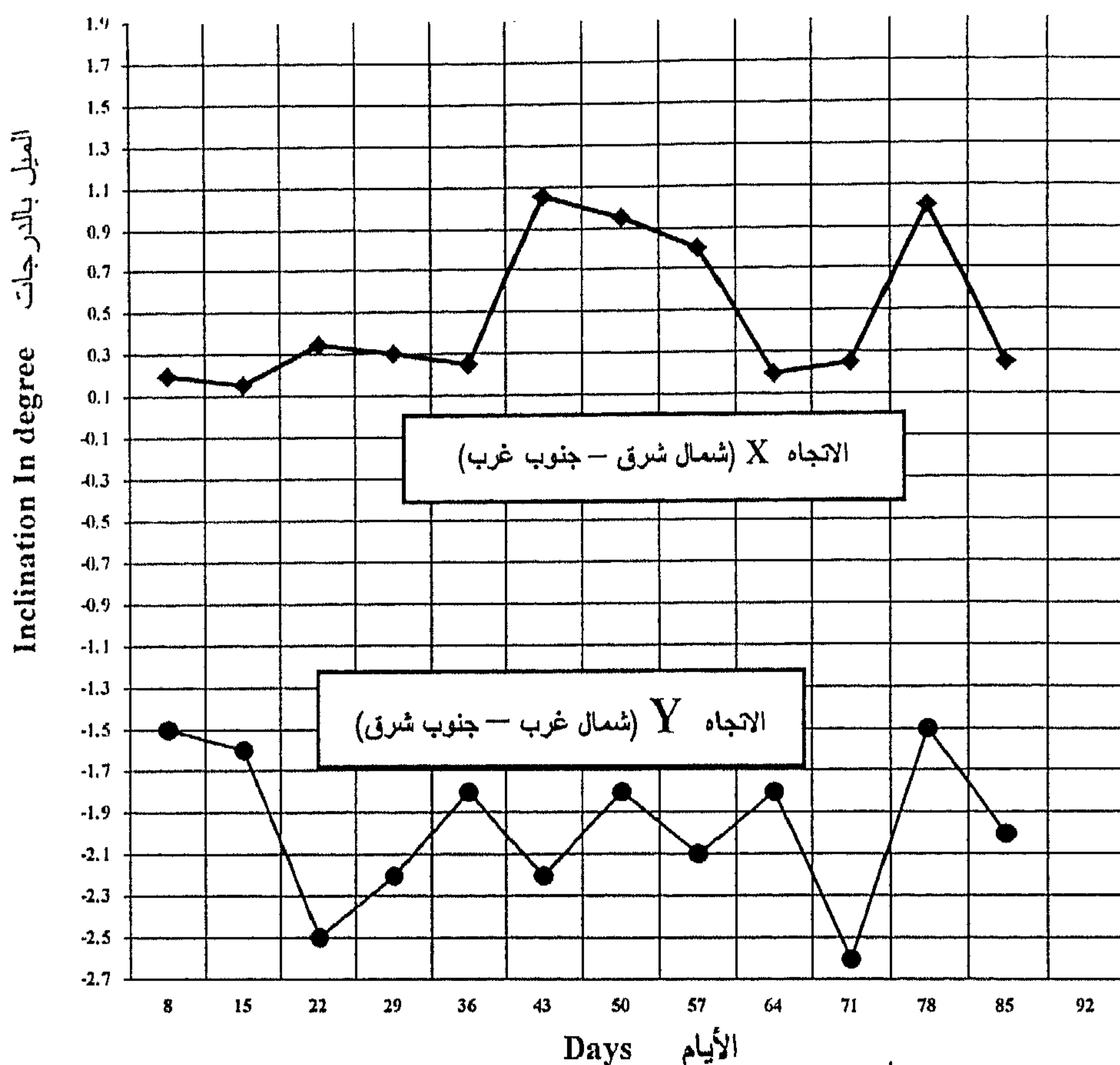
شكل رقم (٣٢) يوضح نتائج مراقبة التغير الديناميكي في الحركة الأفقية لمؤذنة يشبك من مهدي باستخدام جهاز Tiltmeter Differential Micro- Accelerometer
