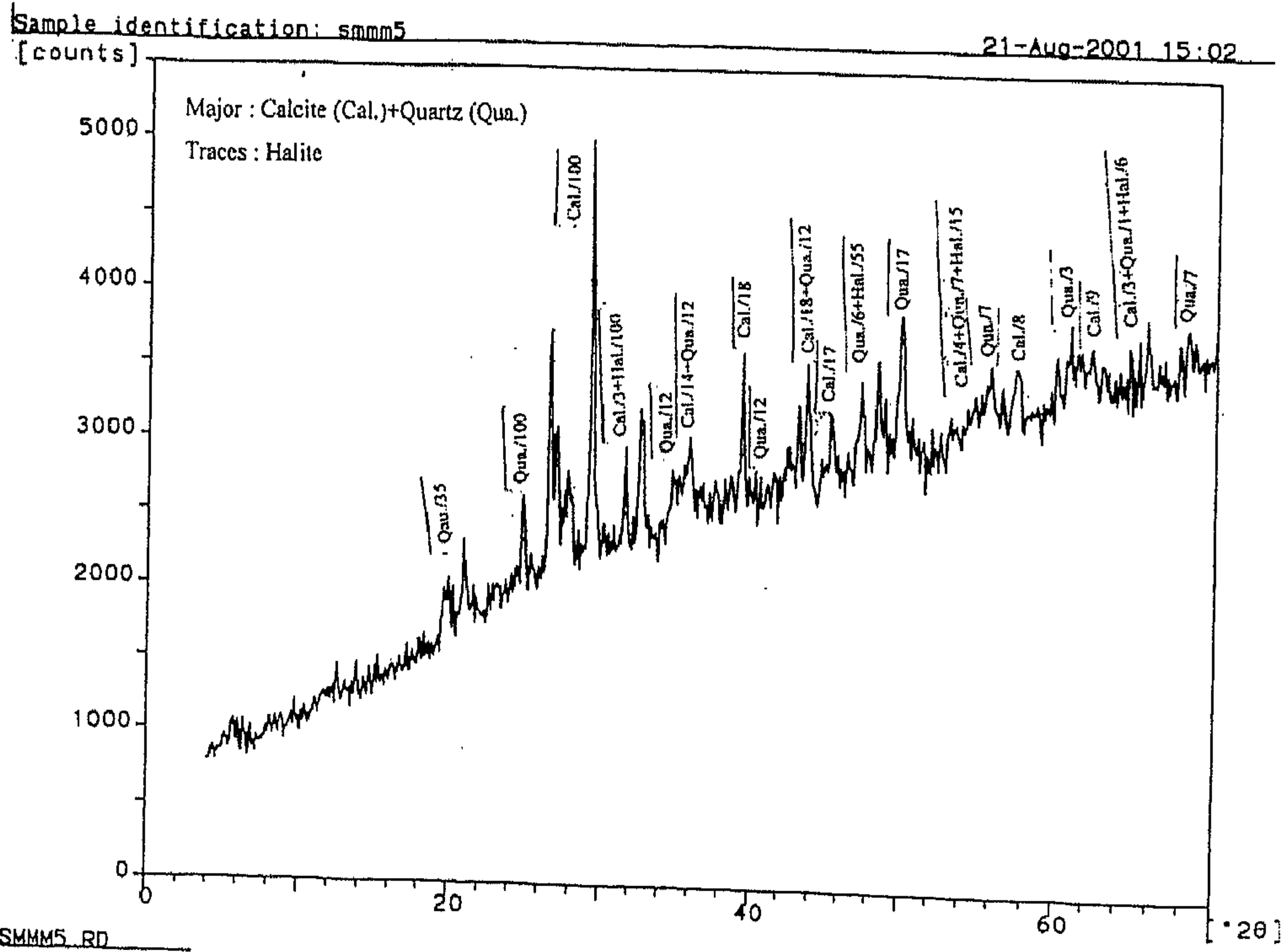
شكل رقم (٣٨) يوضح نمط حيود الأشعة السينية لعينة من مونة الحشو الداخلى بين الأحجار بقاعدة مثذنة يشبك من مهدى
