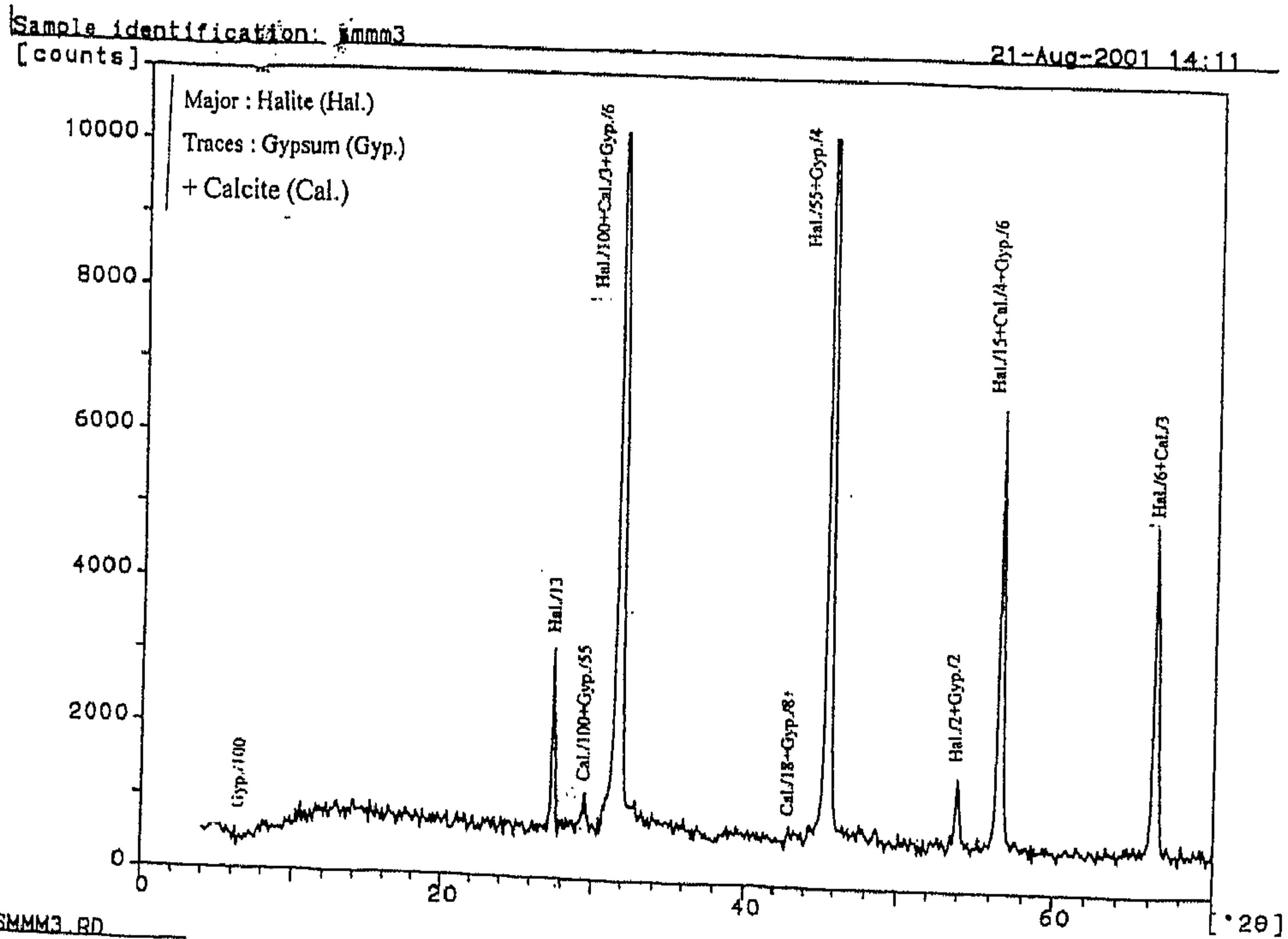
شكل رقم (٣٦) يوضح نمط حيود الأشعة السينية لعينة أملاح أخرى من مئذنة يشبك من مهدى
