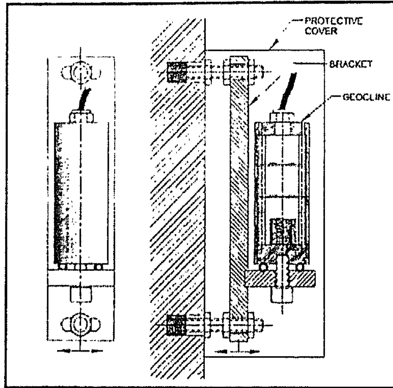
شكل رقم (٣٠) يوضح وحدة قياس الميل Incliner Sensor unit
