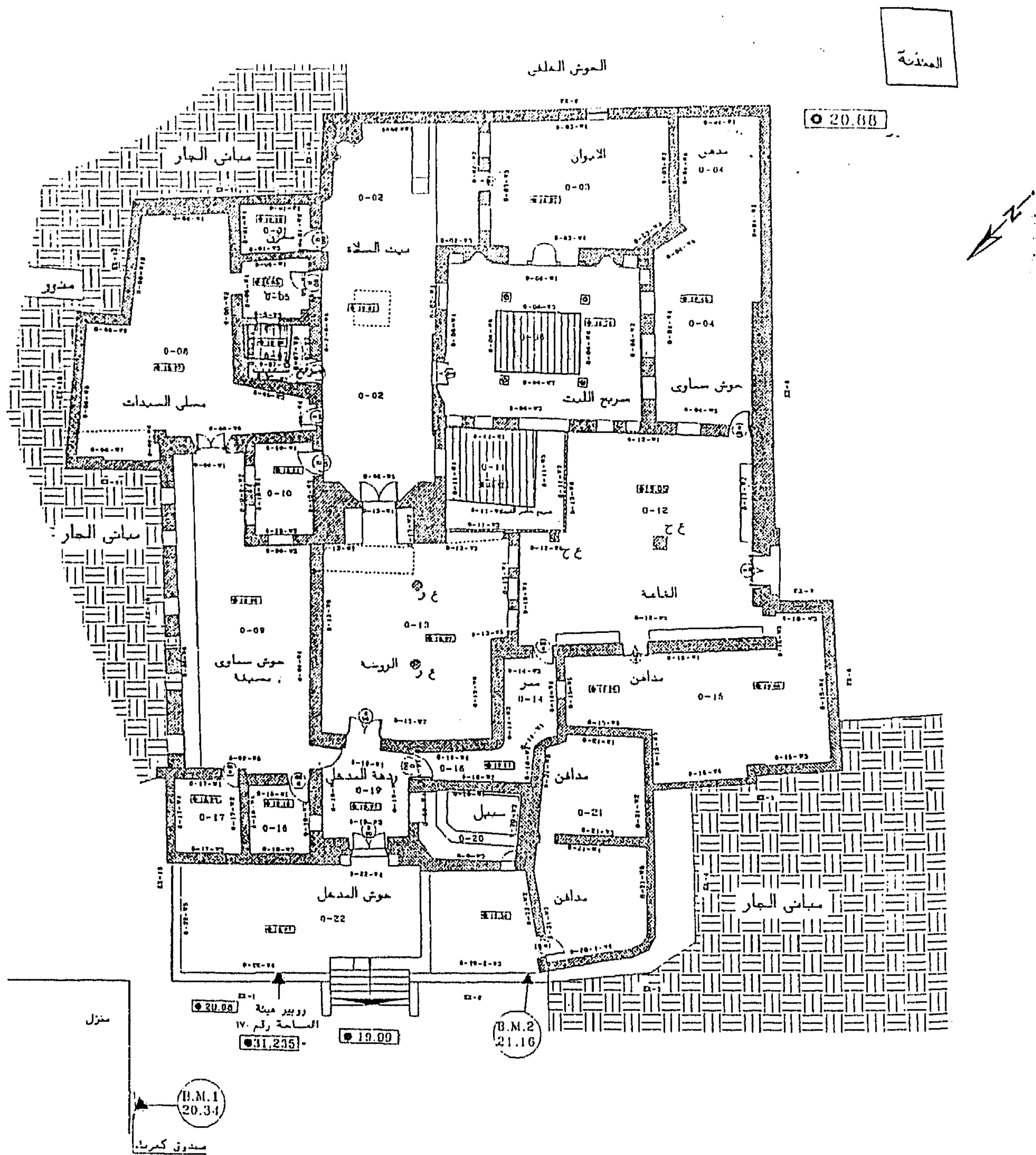
شكل رقم (٢٩) يوضح موقع الروبيرات المساحية بموقع منڈنة يشك من مهدى (عن قطاع المشروعات بالمجلس الأعلى للآثار)
