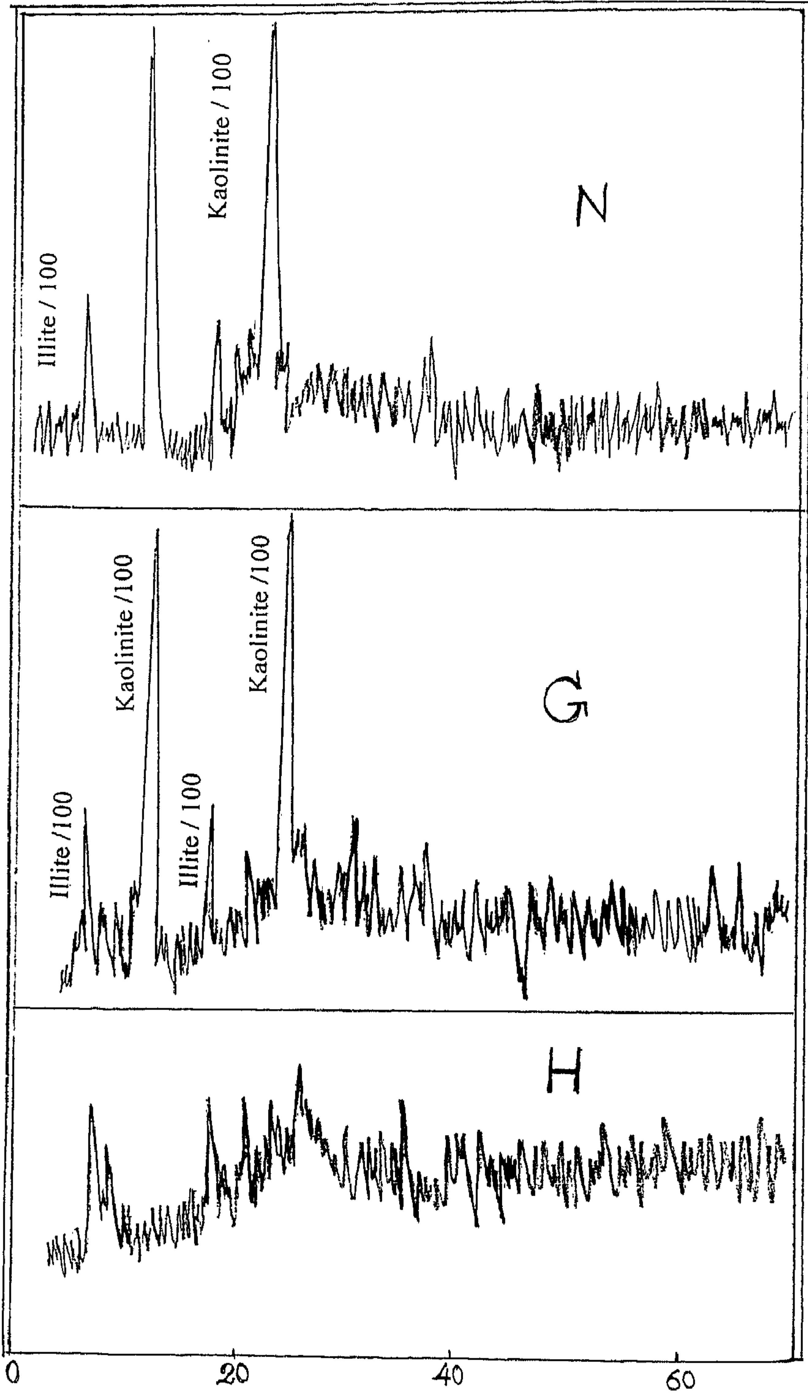
شكل رقم (٤٦) يوضح مقارنة بين أنماط حيود الأشعة السينية لعينة معادن الطفلة التي تم فصلها من التربة بموقع مئذنة يشبك من مهدى وهي تتكون بشكل أساسي من معدنى الأليلت والكاولينيت الذى يختفى بالتسخين.
