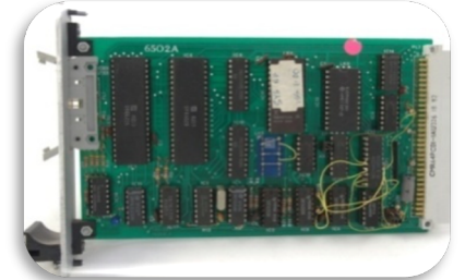
أ / وحدة المعالجة المركزية (المعالج المركزي)
