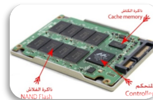
ب / وحدات الذاكرة الذاكرة الرئيسية أو العشوائية RAM الذاكرة المخبأة أو ذاكرة الكاش الذاكرة القرائية فقط
