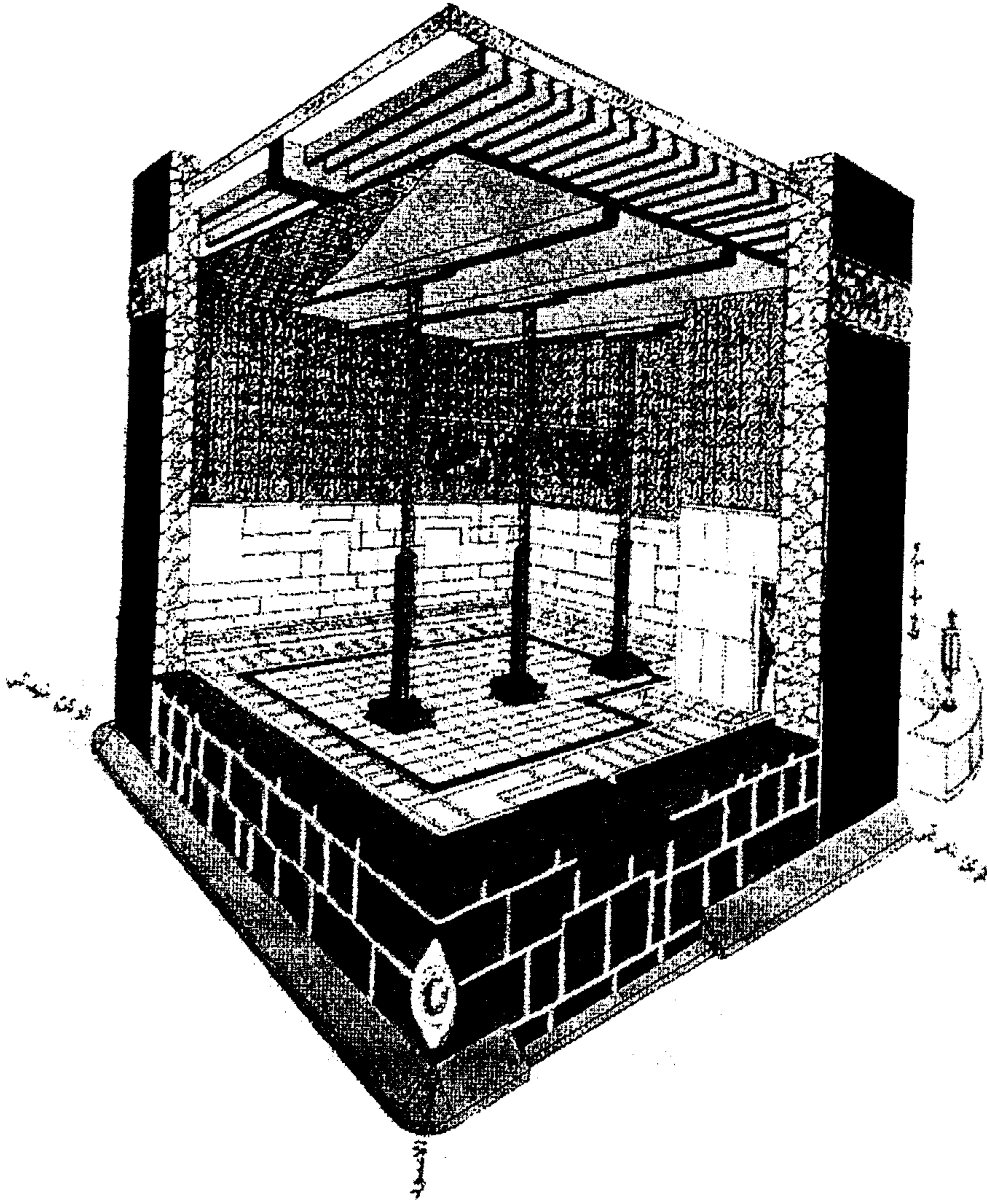
مخطط تفصيلي لداخل الكعبة المشرفة
