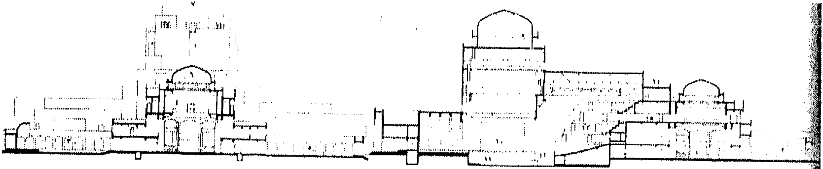
قطاع رأسي عمودي علي المدخل والساحة المكشوفة وقاعة المسرح الرئيسي
