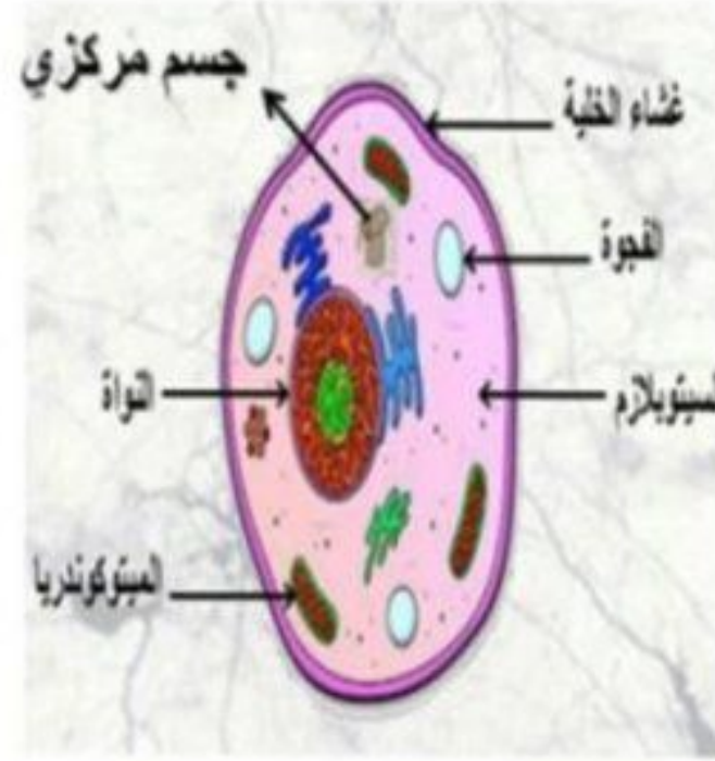
خلية حيوانية
