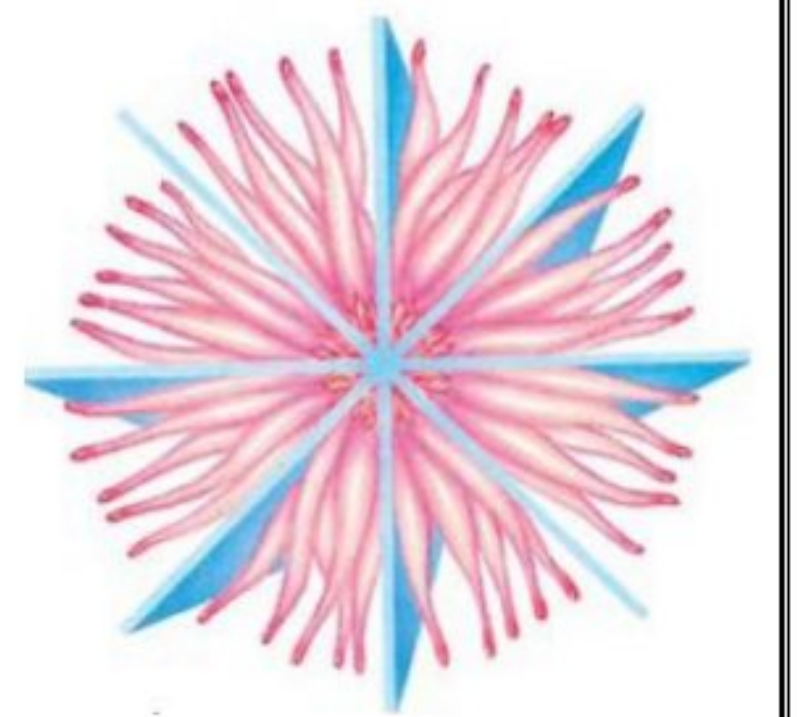
تماثل شعاعي
