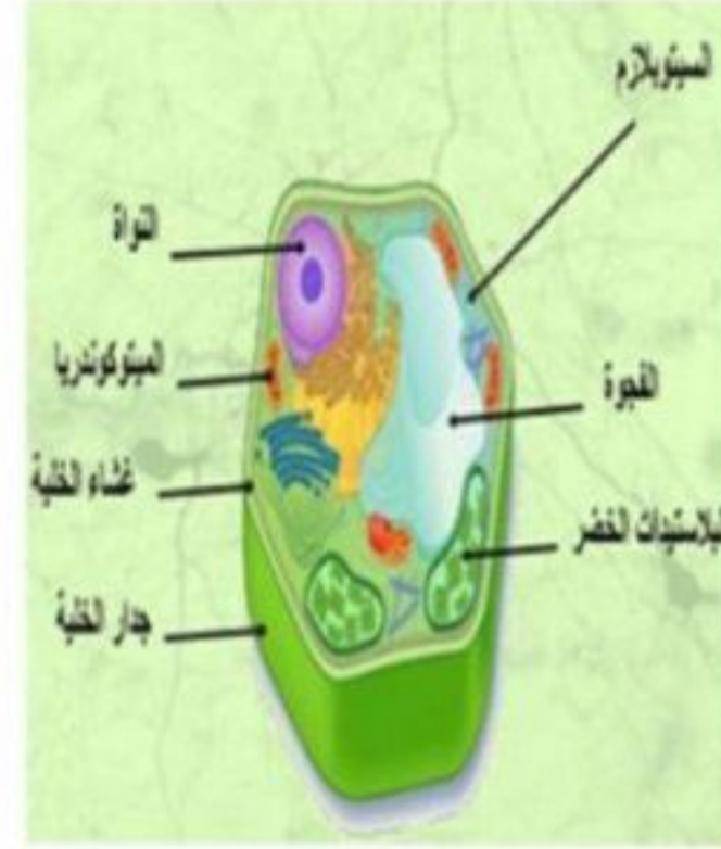
خلية نباتية
