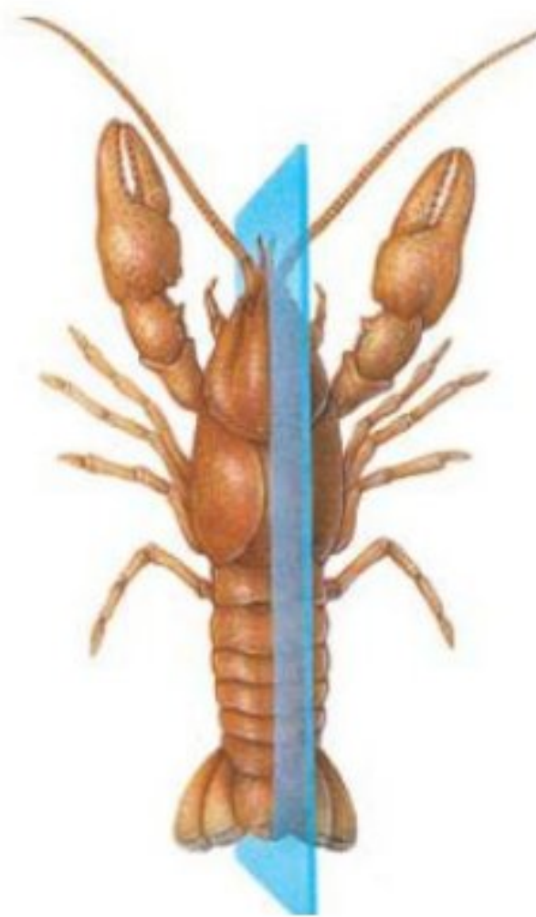
تماثل جانبي
